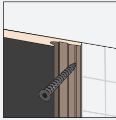
Bevestigen panelen met schroeven, nagels of nieten
